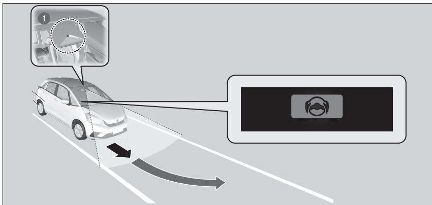
1 Predná širokouhlá kamera: Monitoruje čiary jazdného pruhu
